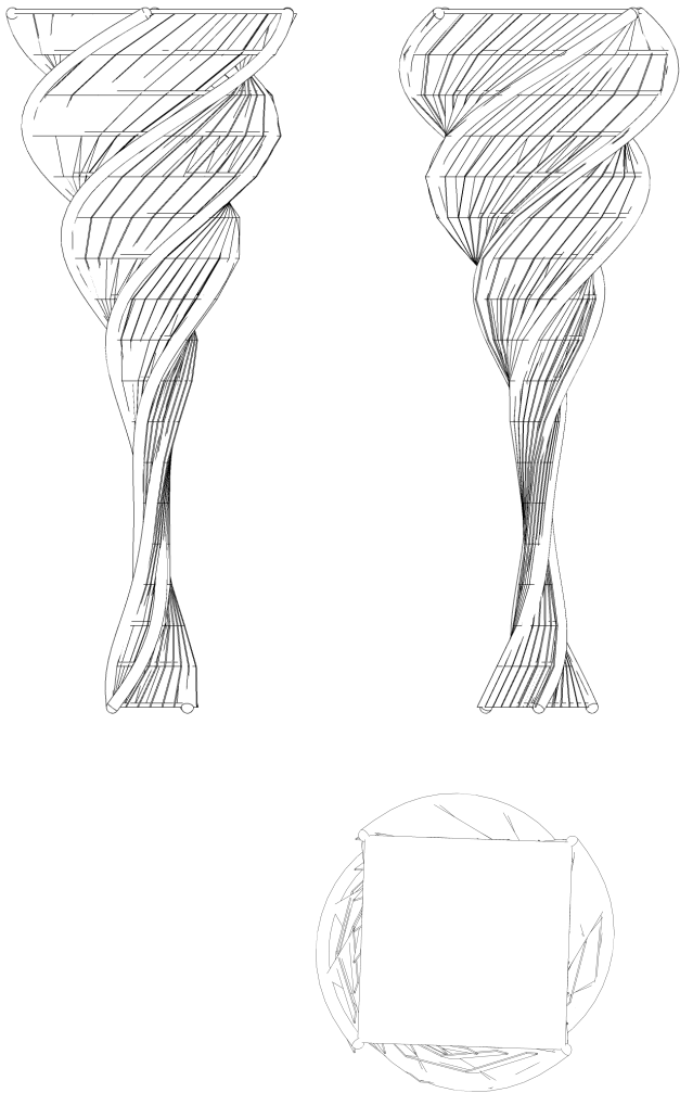
ANSICHTEN UND DRAUFSICHT
